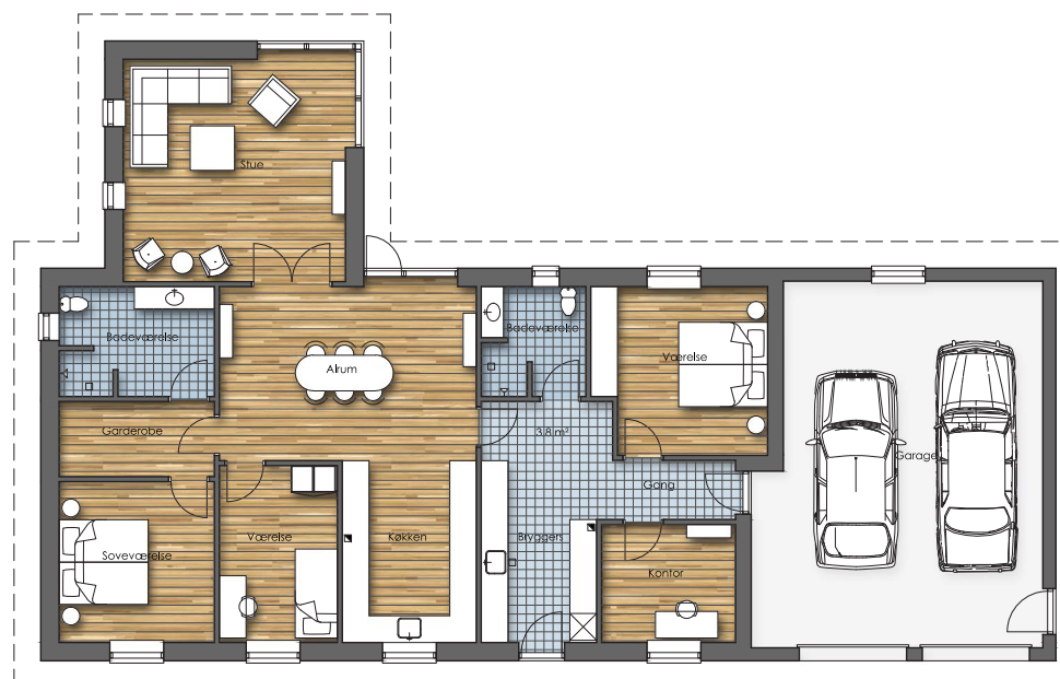
GRUNDPLAN 172 m 2 Beboelse
